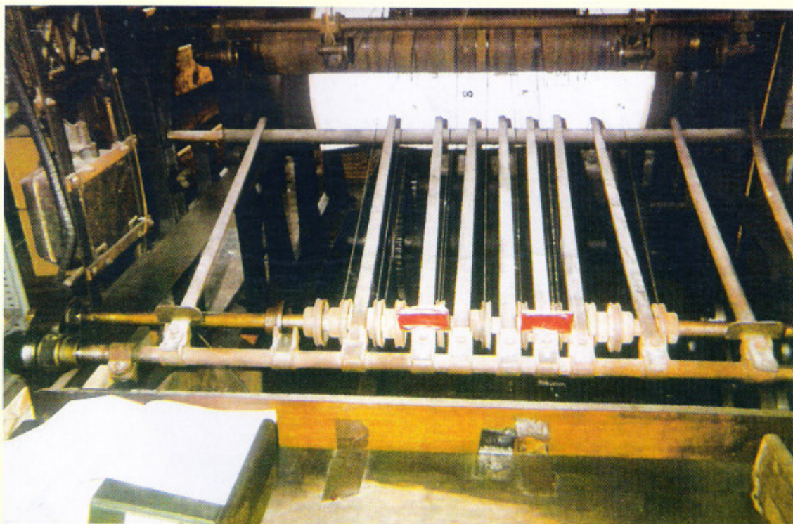
A la sortie de l'impression rotative les feuilles sortent au moyen de lamelles. Photo Lolita JONNIAU.
